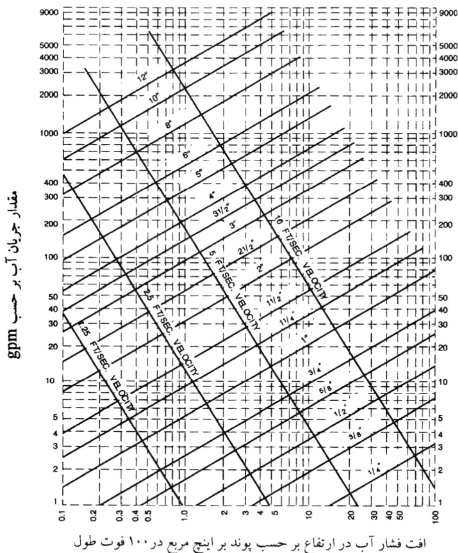
شکل پ - ۱ - ۵ - ۶ (IP) منحنی اندازه‌گذاری لوله‌های مسی نوع L از استاندارد ANSI B ۸۸
